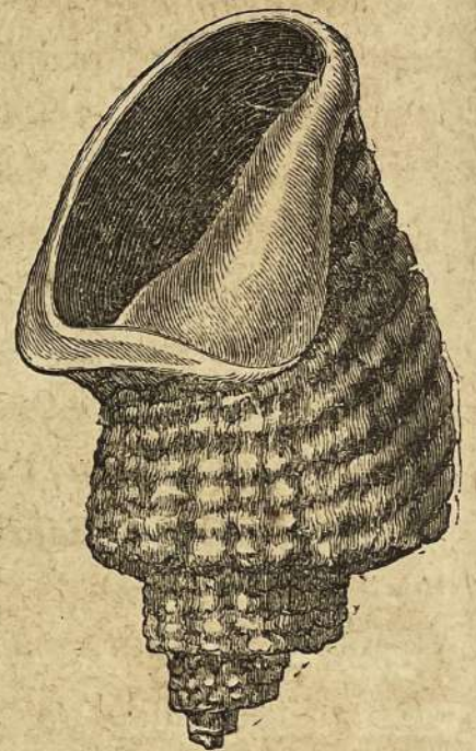
Fig. 88. Acteonina armata Stopp. (Strati d'Esino).
