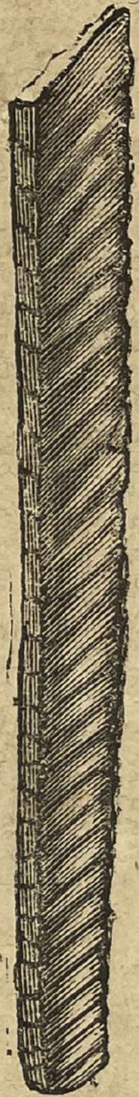
Fig. 74. Baculites neocomiensis d' Orb. (Neocomiano).
