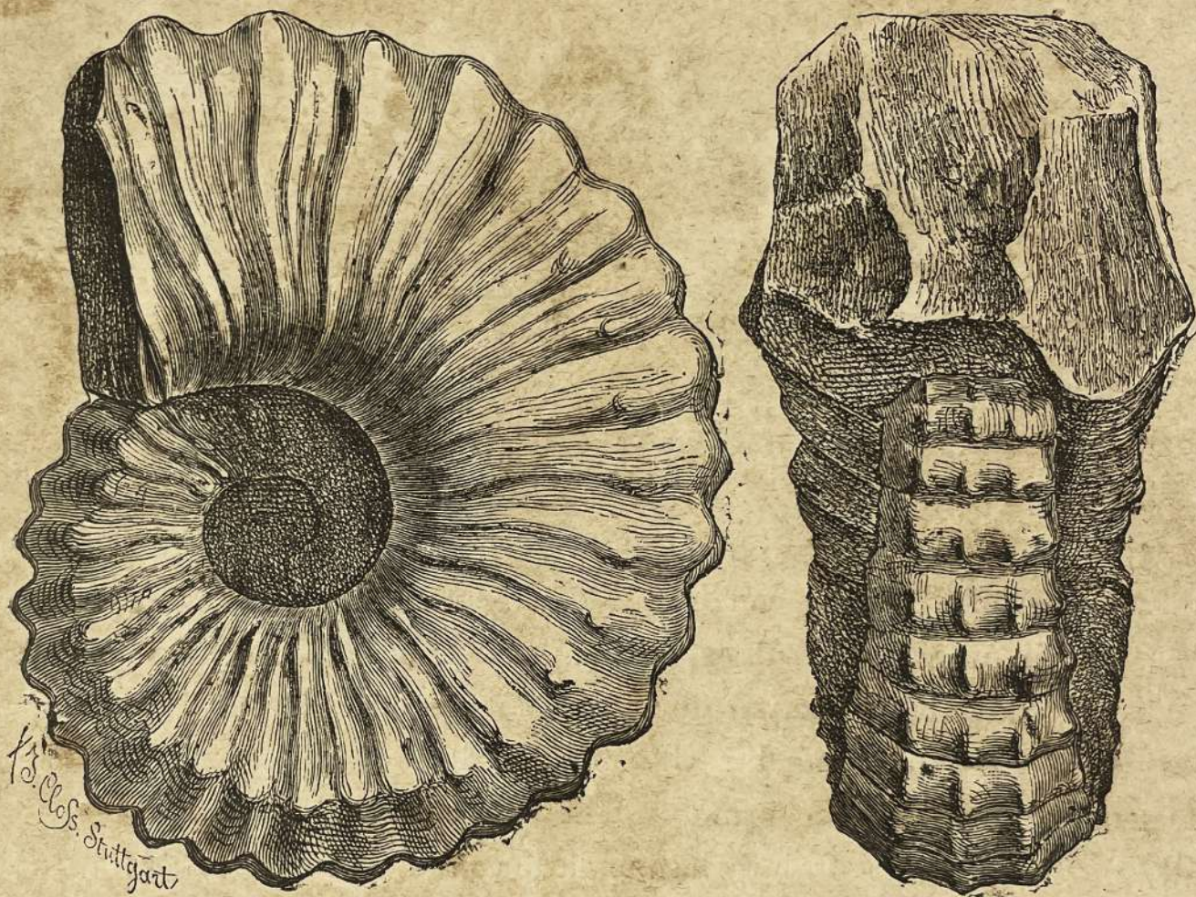
Fig. 71. Ammonites routhomagensis Defr. (Creta superiore).
