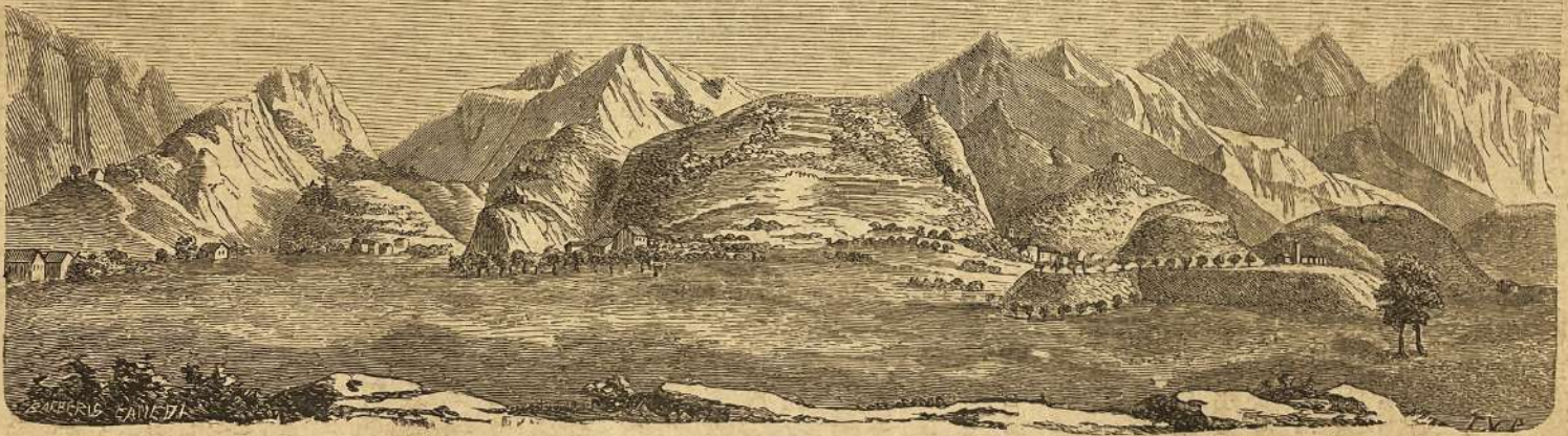
Fig. 139. Colli arrotondati presso Clusone.
